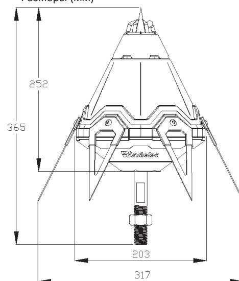
Размеры (мм)
